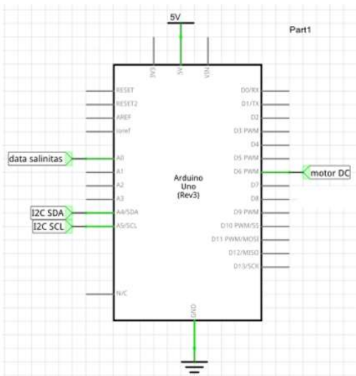
Gambar 2 Rangkaian Arduino Uno R3
