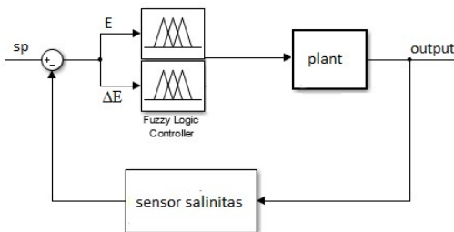
Gambar 9 Blok Diagram Sistem Kontrol Fuzzy
