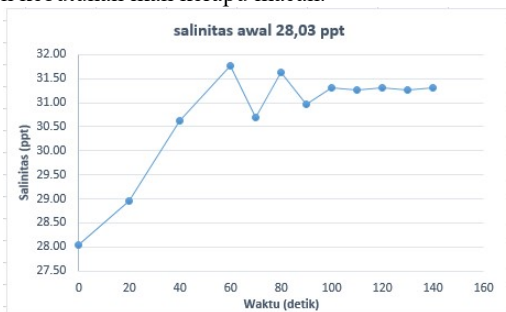
Gambar 14 Perubahan Salinitas pada Kondisi Kedua
