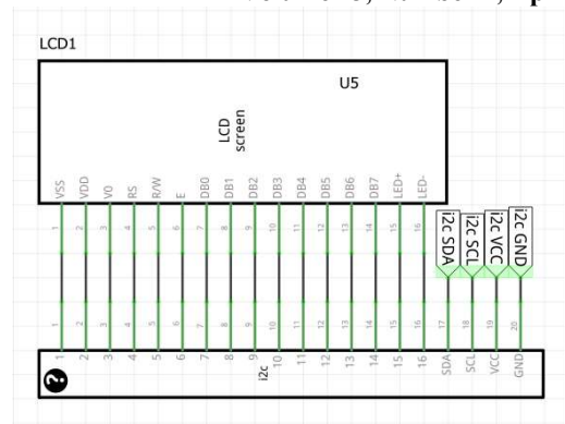
Gambar 3 Rangkaian LCD
