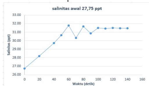
Gambar 12 Perubahan Salinitas pada Kondisi Pertama
