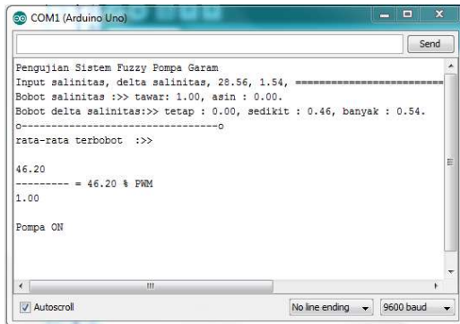
Gambar 11 Hasil pengujian metode fuzzy
